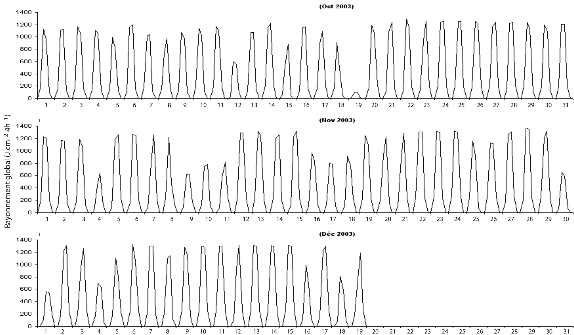
Figure 5. Rayonnement global intégré sur 4h (données Météo-France pour la station du Faubourg Blanchot).
