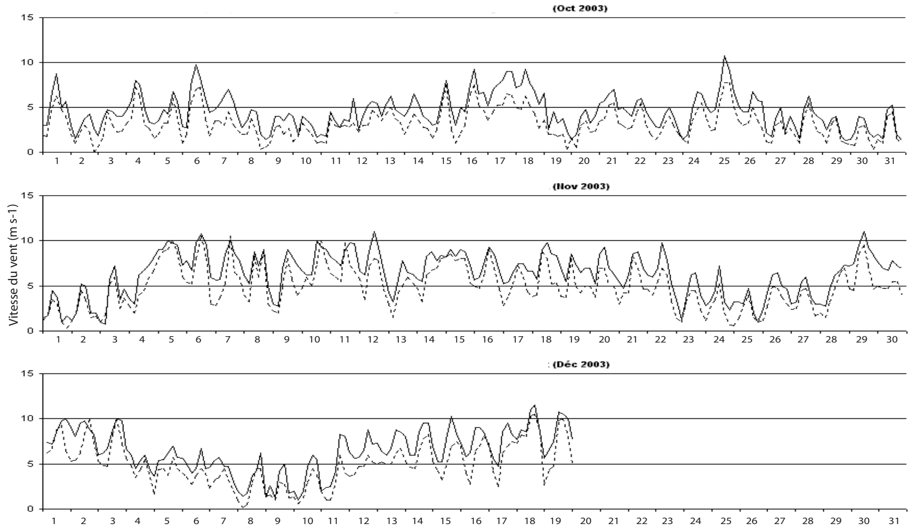
Figure 3. Vitesse du vent moyennée sur 4h (données Météo-France). En pointillé, données de Magenta, en traits pleins, données du Faubourg Blanchot.
