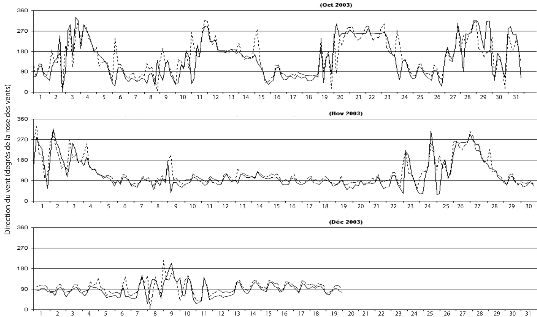
Figure 2. Direction du vent moyennée sur 4h (données Météo-France). En pointillés, données de Magenta, en traits pleins, données du Faubourg Blanchot.
